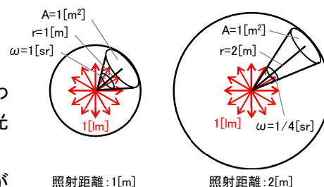
図 8. 照度の計算例
