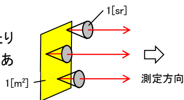
図 10. 輝度の定義
