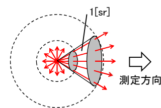
図 5. 光度の定義
