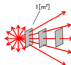
図 7. 照度の定義
