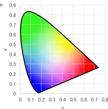
図 13. xy 色度図※3
